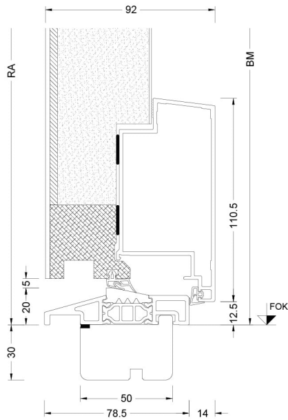
Schnitt unten / Section - bottom
